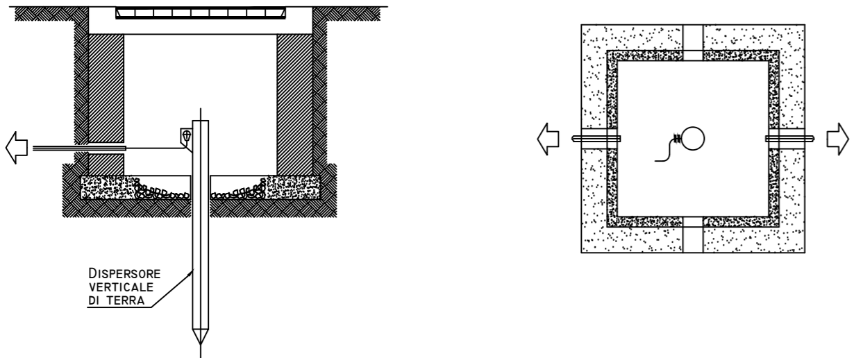
POZZETTO DI TERRA CON DISPERSORE VERTICALE
